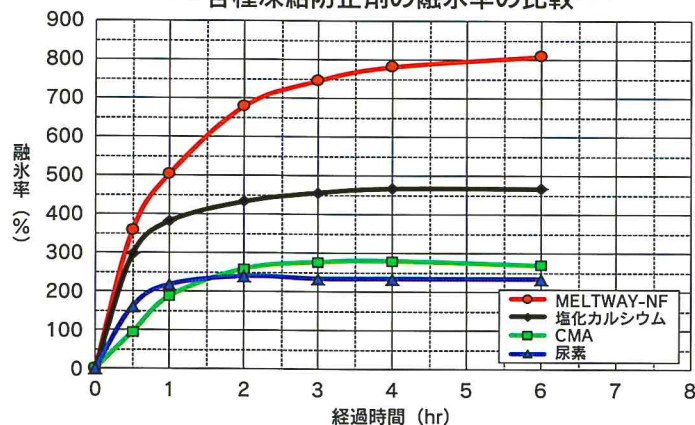
— 各種凍結防止剤の融氷率の比較 —
